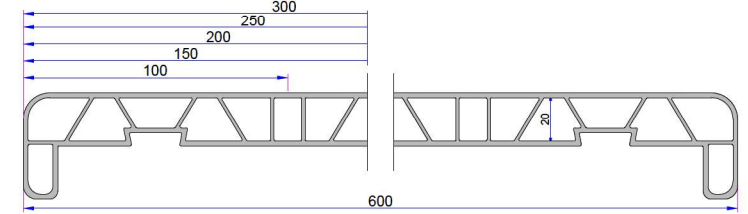
PVC Denizlik Profili (600mm) P.DNZ.01.60.E.600.19
