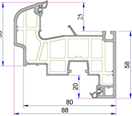
Damlalıklı Kanat Profili P.A.883.2200.600.2.BC.01
