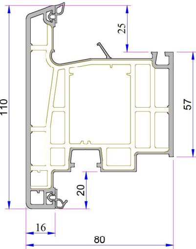
Dışa Açılım Kapı Kanat Profili P.A.883.2101.600.2.BC.01
