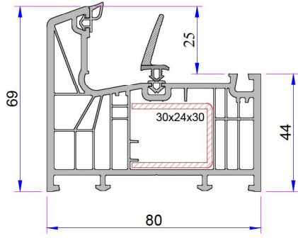
Kasa Profili P.A.883.1000.600.2.BC.01 Destek Sacı (30x24x30)
