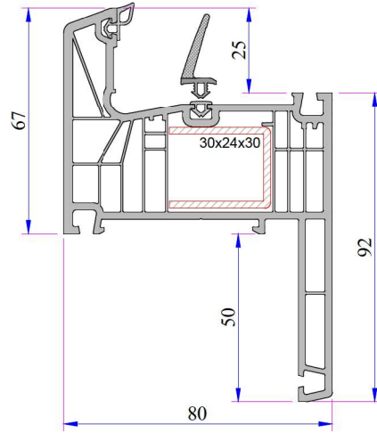
Pervazlı Kasa Profili P.A.883.1200.600.2.BC.01 Destek Sacı (30x24x30)
