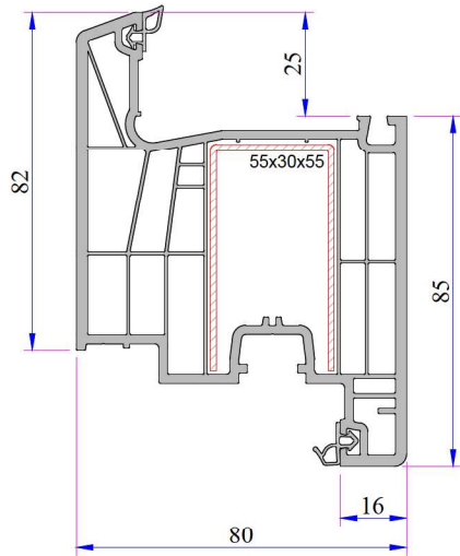
Kapı Kanat Profili P.A.883.2100.600.1.BC.01 Destek Sacı (55x30x55)
