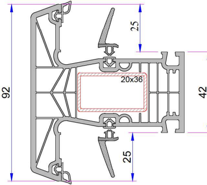
Orta Kayıt Profili P.A.883.3000.600.2.BC.01 Destek Sacı (20x36)
