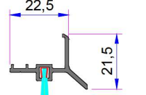
Alm. Eşik Damlalık Profili AD16-057
