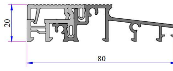
Alm. Yalıtımlı Eşik Profili AD16-090
