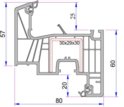
Kanat Profili P.A.883.2000.600.2.BC.01 Destek Sacı (30x29x30)
