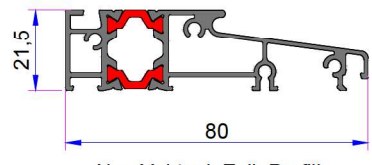
Alm. Yalıtımlı Eşik Profili AD16-056
