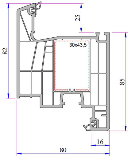
Kapı Kanat Profili (Kutu Destek Sacı) P.A.883.2113.600.1.BC.01 Destek Sacı (11,5x43,5x30x43,5x11,5)
