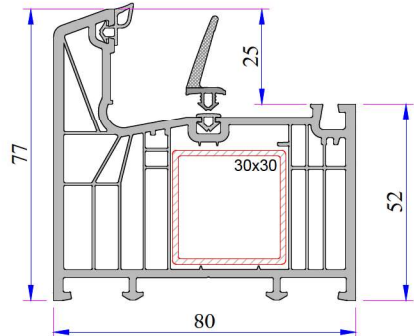
Süper Kasa Profili P.A.883.1001.600.2.BC.01 Destek Sacı (30x30)
