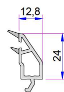
44mm Cam Çıtası P.A.883.4800.600.0.HC
