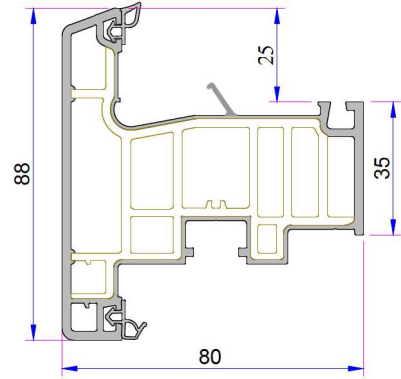
Dışa Açılım Kanat Profili P.A.883.2001.600.2.BC.01
