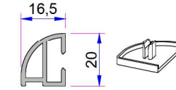
Damlalık Profili P.A.080.5106.600.0.00.19
