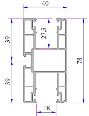
55'lik Lamel Orta Ray Kod: P.A.097.5614.600.0.00.19
