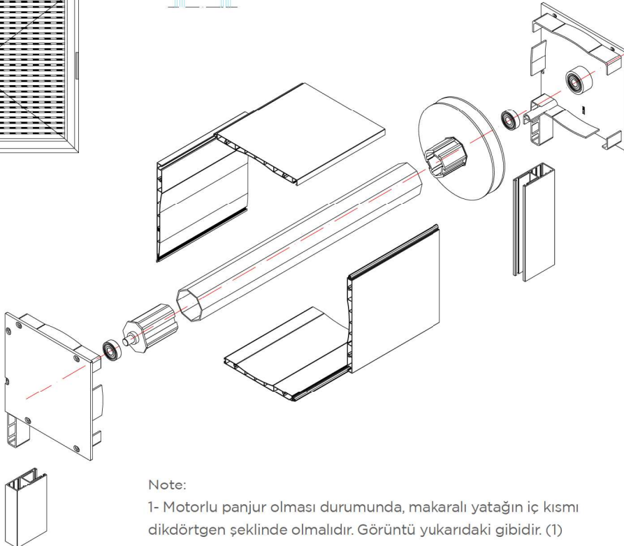
155x155 mm Motorlu Panjur Yan Kapak (Sağ ve Sol ayırılır) Kod: 34019-11050
