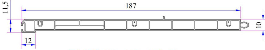
225x225'lik Yalıtımlı Kutu Alt Profili Kod: P.A.097.5612.600.0.00.19
