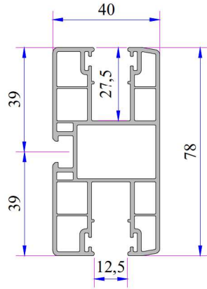
37'lik Lamel Orta Ray Kod: P.A.097.5603.600.0.00.19
