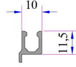
Alm. Tampon Çıtası Kod: 16036.601.5.11.9016
