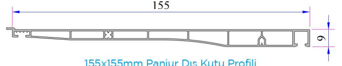
155x155mm Panjur Dış Kutu Profili Kod: P.A.097.5606.600.0.00.19
