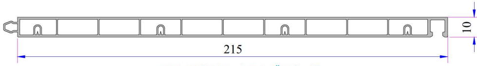
190x225 Yalıtımlı Kutu Üst Profili Kod: P.A.097.5611.600.0.00.19
