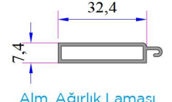
Alm. Ağırlık Laması Kod: 16012.601.5.1.1.9016
