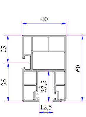
37'lik Lamel Yan Ray Kod: P.A.097.5602.600.0.00.19
