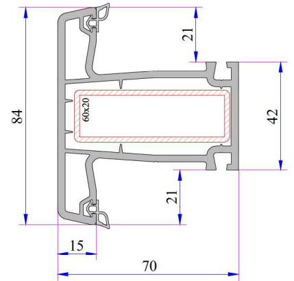
Süper Statik Orta Kayıt Profili Kod: P.A.750.3009.600.0.BC.01
