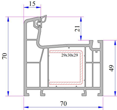
Süper Kasa Profili Kod: P.A.750.1001.600.0.BC.01
