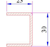
Dışa Açılım Kanat Profili Destek Sacı Kod: 34022-12030
