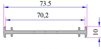
İnce Bağ Profili Kod: P.A.070.5001.600
