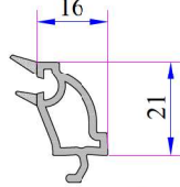
32 mm Dekoratif Contalı Üçlü Cam Çıtası
