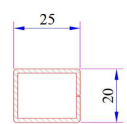
35mm Kasa Yükseltme Profili Destek Sacı Kod: 34022-12104
