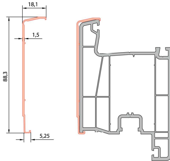
Alüminyum Giydırme Kapı Kanat Profili
