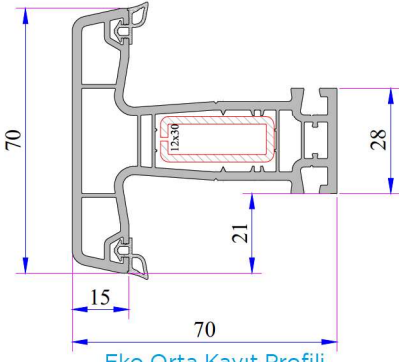
Eko Orta Kayıt Profili
