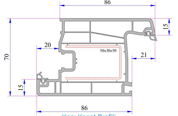
Kapı Kanat Profili
