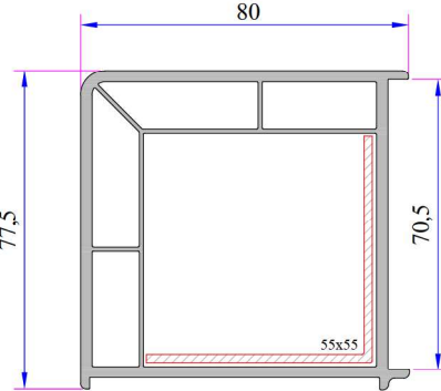
90° Köşe Profili Kod: P.A.070.5100.600.0.00.19
