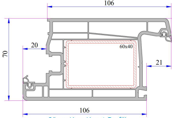
Süper Kapı Kanat Profili
