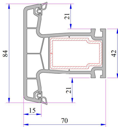
Statik Orta Kayıt Profili Kod: P.A.750.3007.600.0.BC.01
