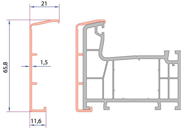
Alm. Giydırme Normal Kasa Profili
