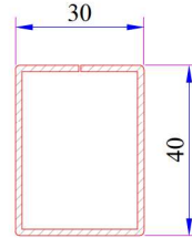
100mm Kasa Yükseltme Profili Destek Sacı Kod: 34022-12120
