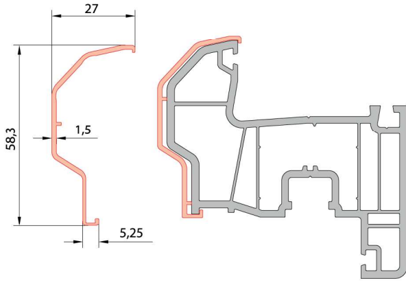
Alüminyum Giydırme Damlalıklı Kanat Profili
