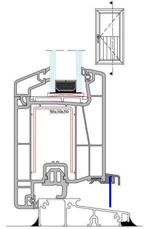
Alüminyum Eşikli Kasa - Kapı Kanat Montajı
