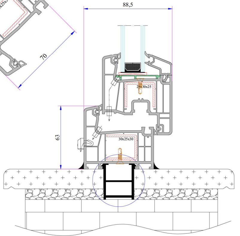
Kasa Montaj Profili Kullanım Detayı
