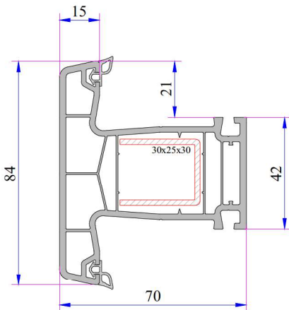
Orta Kayıt Profili Kod: P.A.750.3000.600.0.BC.01
