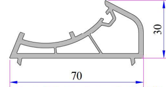
Açılı Dönüş Adaptör Profili Kod: P.A.070.5104.600.0.00.19
