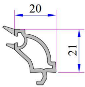
28 mm Dekoratif Contalı Çift Cam Çıtası
