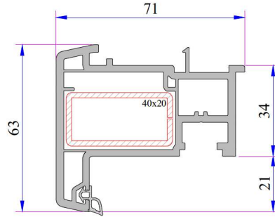
Statik Hareketli Orta Kayıt Profili (Tırnaklı)
