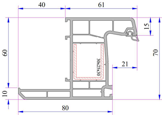
Pervazlı Kasa Profili Kod: P.A.750.1200.600.0.BC.01
