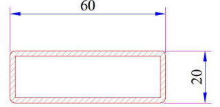
Statik Orta Kayıt Profili Destek Sacı Kod: 34022-12106
