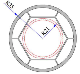
Açılı Dönüş Borusu Ø70mm Kod: P.A.070.5106.600
