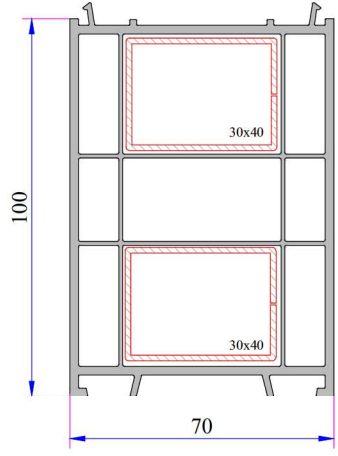
100mm Kasa Yükseltme Profili Kod: P.A.070.5302.600.0.00.19
