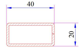
Statik Hareketli Orta Kayıt Profili Destek Sacı Kod: 34022-12114
