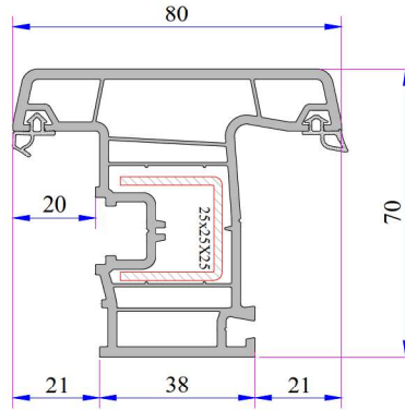
Dışa Açılım Kanat Profili Kod: P.A.750.2001.600.0.BC.01
