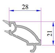
20 mm Dekoratif Contalı Çift Cam Çıtası
