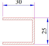
Kasa-Pervazlı Kasa-Orta Kayıt Profili Destek Sacı Kod: 34022-12004
