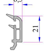
42 mm Contalı Üçlü Cam Çıtası
