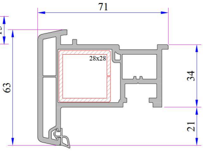
Hareketli Orta Kayıt Profili
