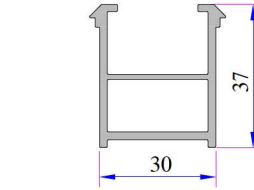
Kasa Montaj Profili Kod: P.A.060.5301.600.0.00.19
