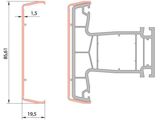
Alüminyum Giydırme Orta Kayıt Profili
