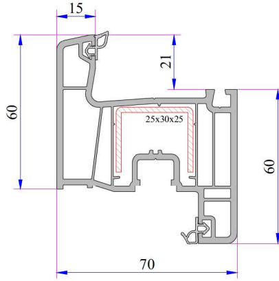
Kanat Profili Kod: P.A.750.2000.600.0.BC.01
