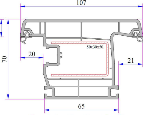
Dışa Açılım Kapı Kanat Profili
