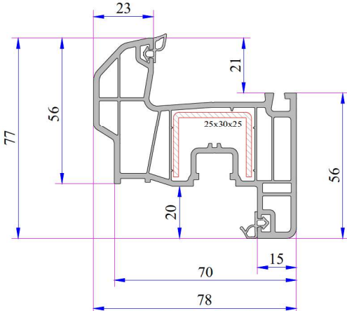
Damlalıklı Kanat Profili (6 Odacıklı) Kod: P.A.750.2205.600.0.BC.01
