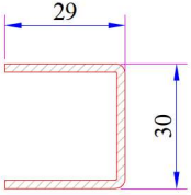
Süper Kasa Profili Destek Sacı Kod: 34022-12002
