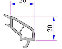
28 mm Contalı Çift Cam Çıtası
