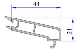
4-6 mm Contalı Tek Cam Çıtası
