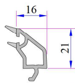
32 mm Contalı Üçlü Cam Çıtası
