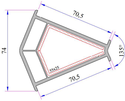
135° Köşe Profili Kod: P.A.070.5102.600.0.00.19
