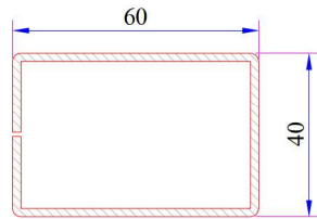
Süper Kapı Kanat - Dışa Açılım Süper Kapı Kanat Profili Destek Sacı Kod: 34022-12110
