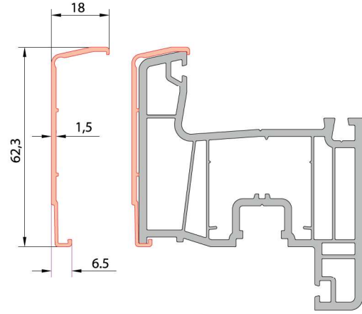
Alüminyum Giydırme Normal Kanat Profili
