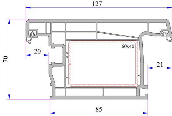
Dışa Açılım Süper Kapı Kanat Profili
