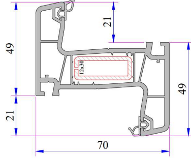
Dışa Açılım Orta Kayıt Profili
