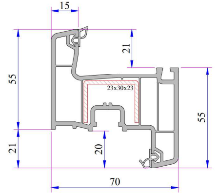
24 Aks Kanat Profili Kod: P.A.750.2003.600.0.BC.01
