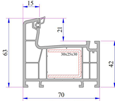
Kasa Profili Kod: P.A.750.1000.600.0.BC.01
