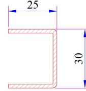
Kanat-Damlalık Kanaat Profili Destek Sacı Kod: 34022-12025
