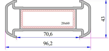
Kalın Bağ Profili Kod: P.A.070.5000.600.0.00.19
