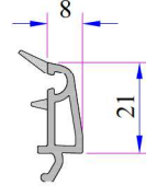
40 mm Contalı Üçlü Cam Çıtası
