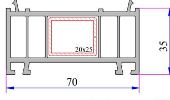
35mm Kasa Yükseltme Profili Kod: P.A.070.5300.600.0.00.19
